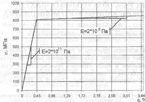
Рис. 2. Зависимость напряжения в материалах цилиндра от относительной деформации
