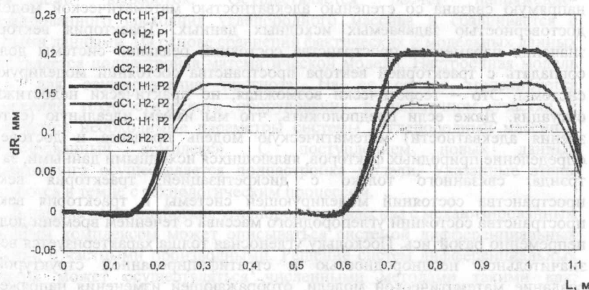
Рис. 3. Радиальные деформации цилиндра при: d_{C1}=0,0225 м; d_{C2}=0,03 м; H_1=0,893 м; H_2=0,445 м; P_1=50 МПа; P_2=75 МПа
