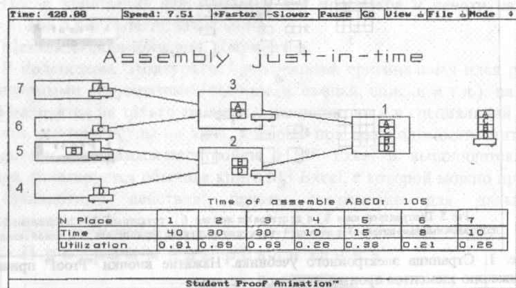
Рис. 3. Кадр компьютерной анимации сборочного производства в режиме "Just-In-Time": вводится случайное время сборочных операций, после имитации отображается процесс сборки и оценивается степень использования сборочных участков
