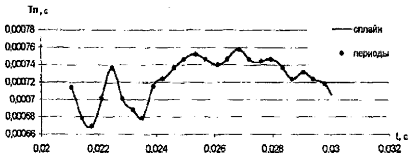
Рис. 2. Аппроксимирующие функции значений периодов T_p по времени t .
