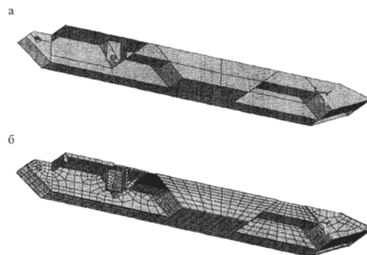
Рис. 3. Модель верхняка крепи 1М130: а) геометрическая модель; б) конечно-элементная модель
