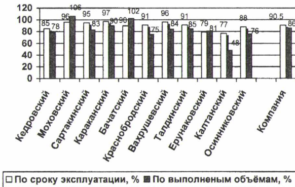
Рис. 1. Износ экскаваторного парка по сроку эксплуатации и выполненным объемам на предприятиях ОАО УК «Кузбассразрезуголь» на 1 января 2005 г.
