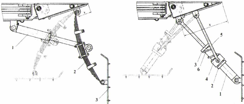
Рис. 1. Активные устройства крепления забоя УКЗ-1 и УКЗ-2
