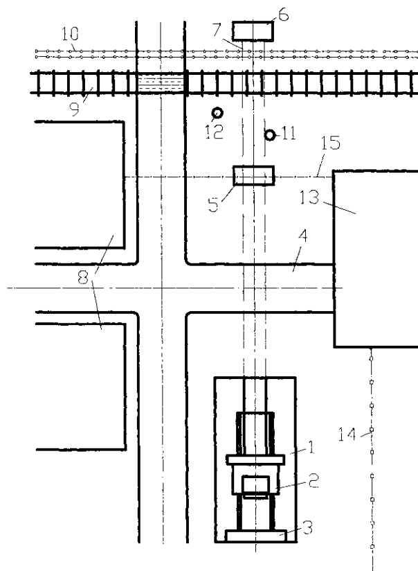
Рис. 1. Схема расположения оборудования и коммуникаций: 1 – рабочий котлован; 2 – бурошнековая машина; 3 – упорная плита; 4 – технологическая дорога; 5 – промежуточный котлован; 6 – приемный котлован; 7 – прокладываемая коммуникация; 8 – складские помещения; 9 – железнодорожный путь; 10 – эстакада с коммуникациями; 11, 12 – опоры ЛЭП; 13 – столярный цех; 14 – ограждение; 15 – действующая канализация
