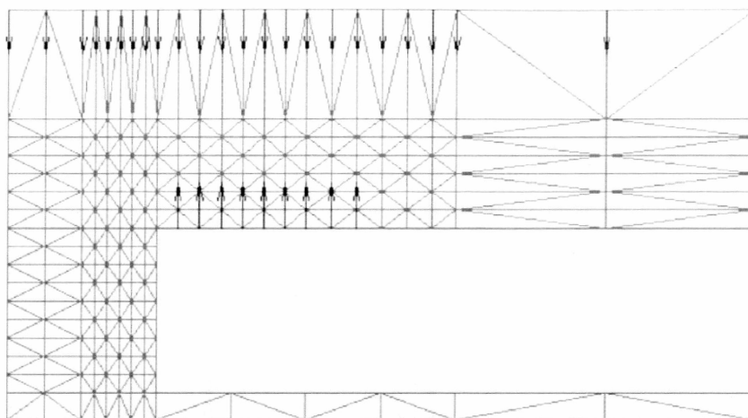
Рис. 1. Сетка конечных элементов и схема приложения нагрузки на модель
