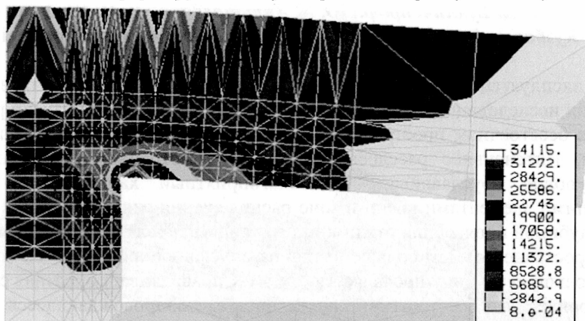
Рис. 2. Распределение напряжений в массиве горных пород вблизи забоя
