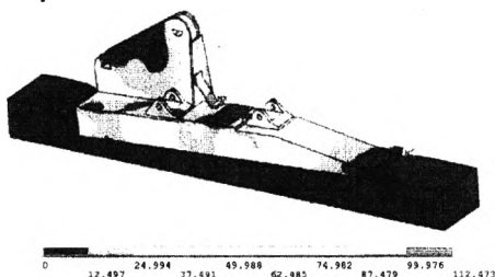
Рис. 1. Напряжённо-деформированное состояние модели основания и почвы
