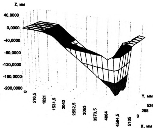
Рис. 2. Распределение вертикальных деформаций поверхности почвы
