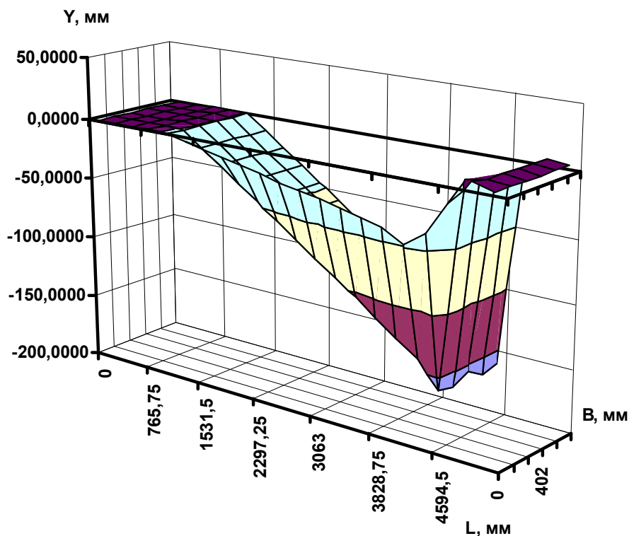
Рис.3. Распределение вертикальных деформаций по поверхности почвы
