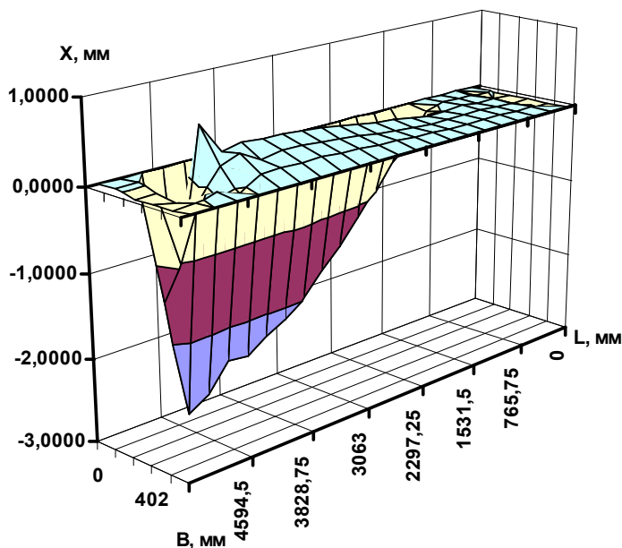
Рис.4. Распределение горизонтальных деформаций по поверхности почвы
