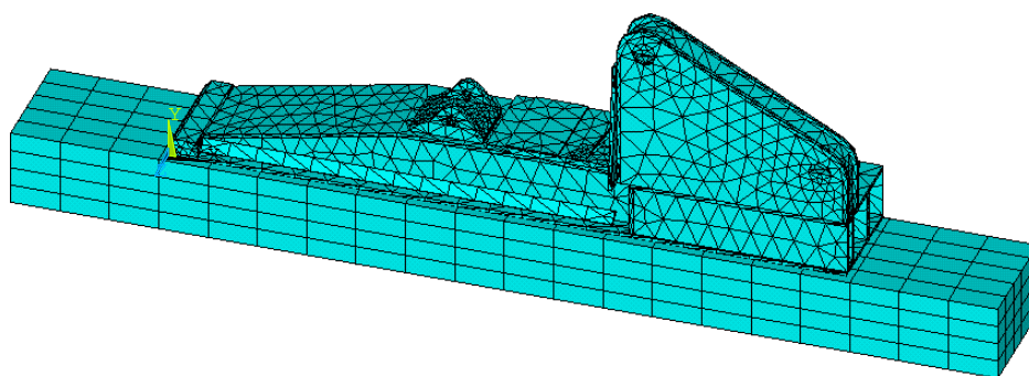
Рис. 1. Конечно-элементная модель основания и почвы
