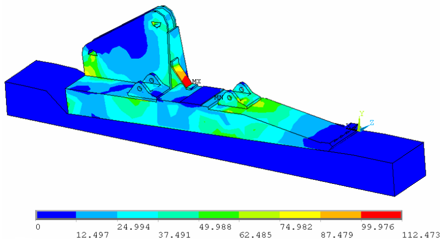
Рис. 2. Напряжённо-деформированное состояние модели основания и почвы
