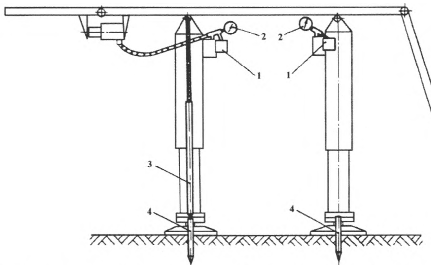
Рис. 1. Схема снятия замеров и расположение приборов на измерительной секции
