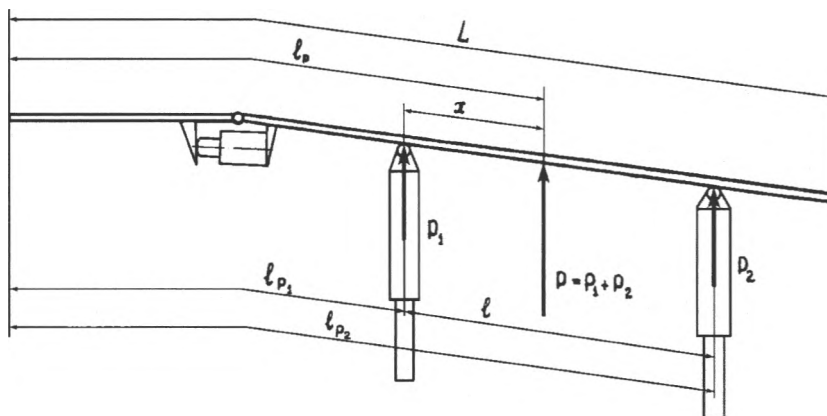
Рис. 2. Схема верхняка
