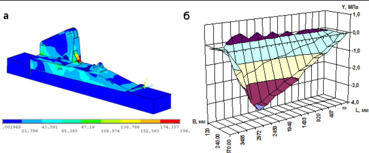
Рис. 2. Напряженно-деформированное состояние модели модернизированного основания крепи 2М142 при взаимодействии с почвой (а) и распределение вертикальных напряжений по поверхности почвы (б) (L и B – длина и ширина основания)
