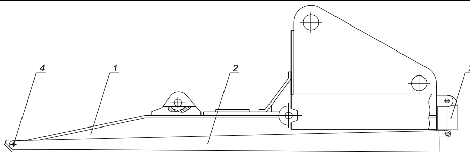
Рис. 1. Модернизированное основание крепи 2М142
