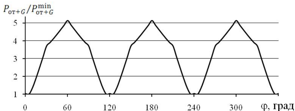
Рис. 3. Колебания отклоняющей силы с учетом силы тяжести в зависимости от угла поворота расширителя \phi при \alpha = 0^\circ
