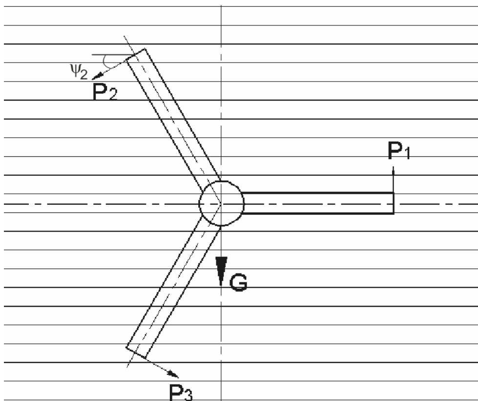
Рис. 1. Схема расположения расширителя относительно линий напластования
