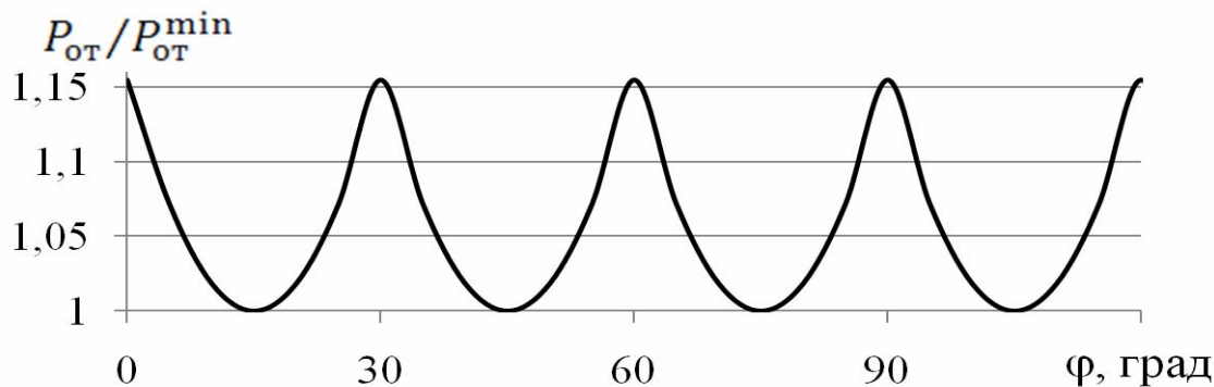
Рис. 2. Колебания отклоняющей силы в зависимости от угла поворота расширителя \phi при \alpha = 0^\circ
