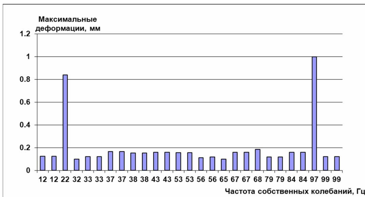
Рис. 2. Максимальные деформации рабочего цилиндра при различных частотах собственных колебаний
