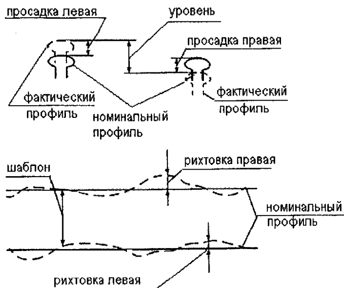
Рис. 2. Параметры отклонения рельсовой колеи от номинального профиля
