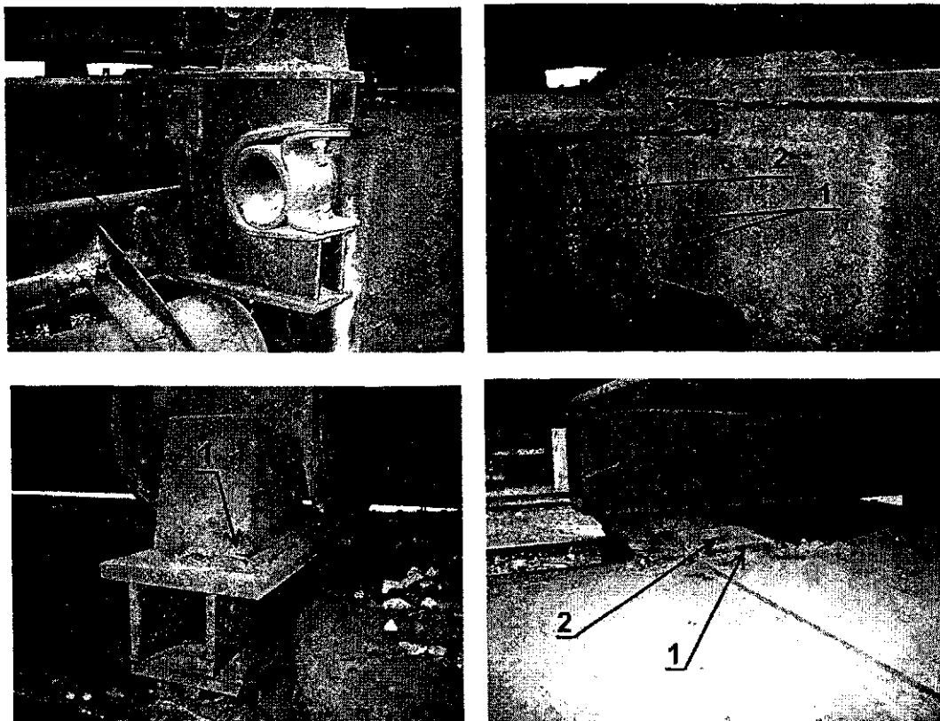
Рис. 1. Примеры устранения трещиноподобных дефектов в рамах думпкаров: 1 – сварной шов; 2 – ремонтная заплата
