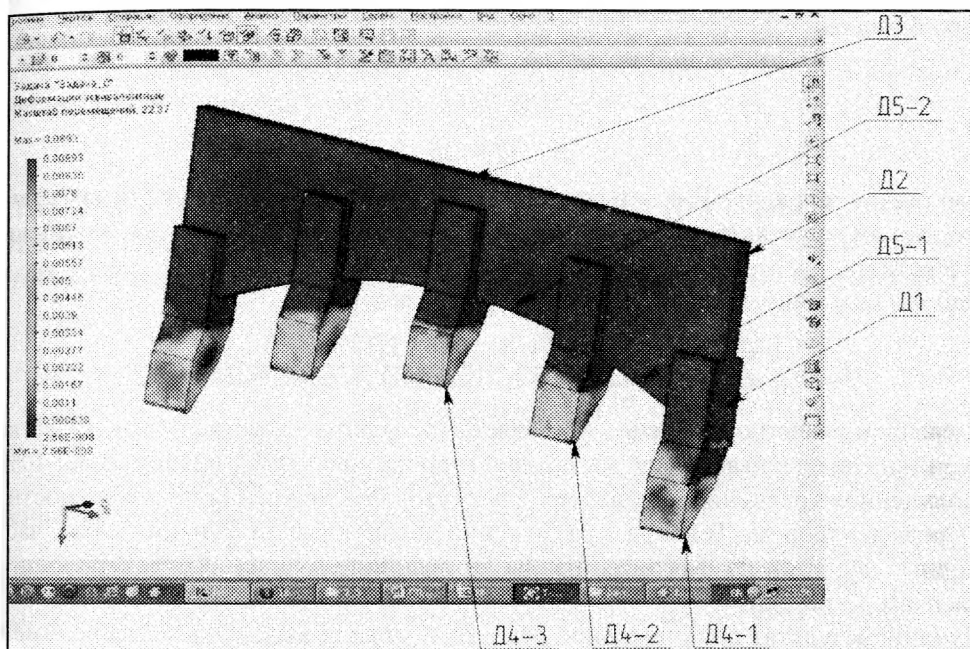
Рисунок 1 – Расстановка датчиков
