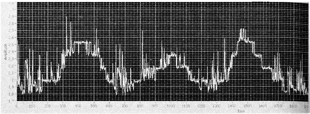
Рис. 2. Фактическая пульсация давления в напорной магистрали гидросистемы при работе трех плунжеров насоса Н403У
