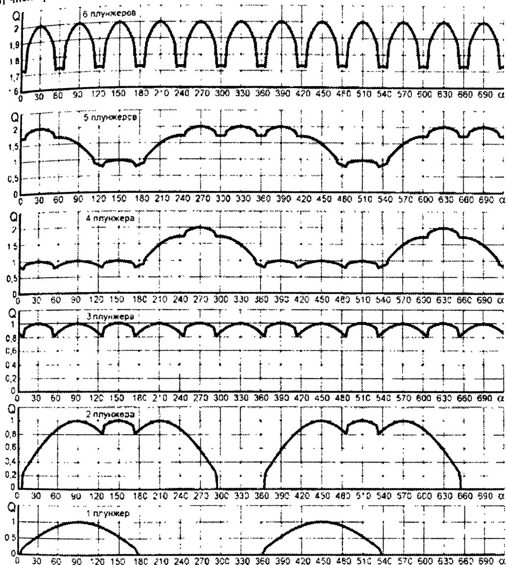
Рис. 1. Графики подачи многопоточного насоса типа Н403У при изменении числа работающих плунжеров от шести до одного
