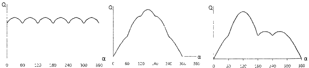
Рис 3. Теоретические графики подачи насоса Н403У при различных схемах включения трех плунжеров
