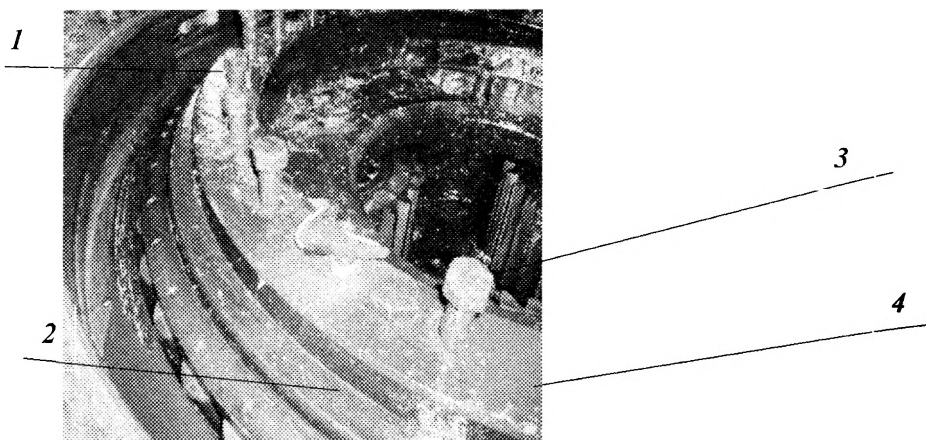
Рис. 3. Мотор-колесо БелАЗа-75131 с установленным датчиком: 1 – редуктор мотор-колесо; 2 – подшипник; 3 – датчик; 4 – упорное кольцо
