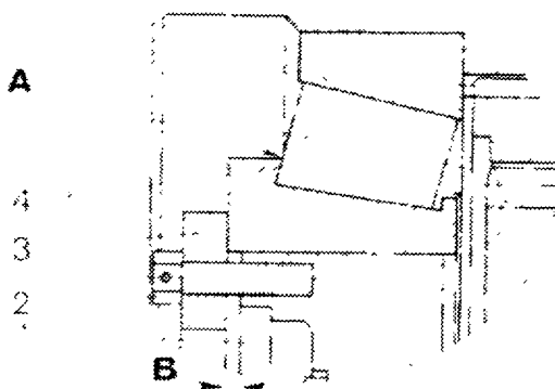
Рис. 6. Проверка зазоров: 1 – корпус редуктора, 2 – болт регулировочный; 3 – кольцо упорное, 4 – подшипник; А – место установки щупа; В – зазор
