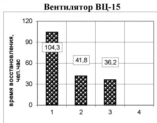
Рисунок 3. Трудоемкость восстановления работоспособности
