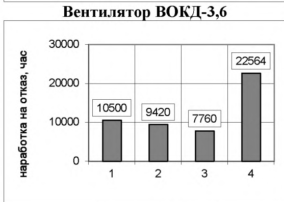
Рисунок 2. Нарботка на отказ механического оборудования
