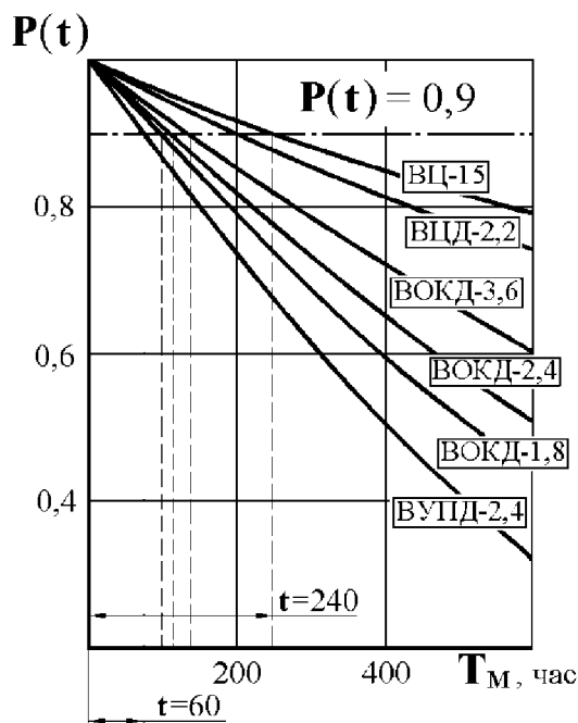
Рисунок. 1. Вероятность безотказной работы ВГП на шахтах Кузбасса
