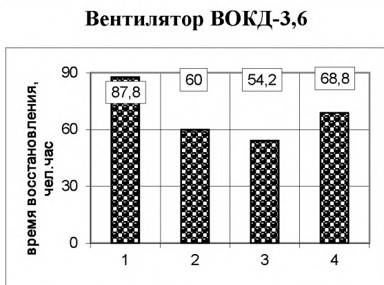
Рисунок 3. Трудоемкость восстановления работоспособности
