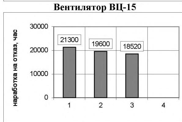
Рисунок 2. Нарботка на отказ механического оборудования
