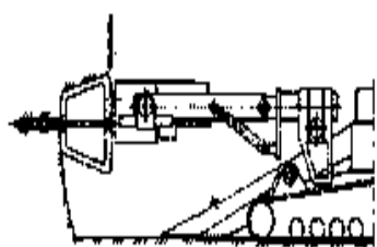
Рис.2. Коронка со сквозным каналом
