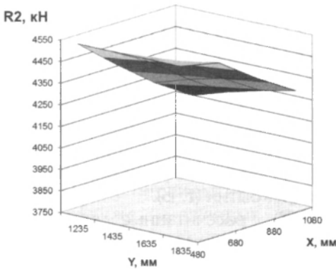
Рис. 3. Реакции R_1 и R_2 в зависимости от расположения точек крепления углового домкрата ( X и Y на рис. 2)
