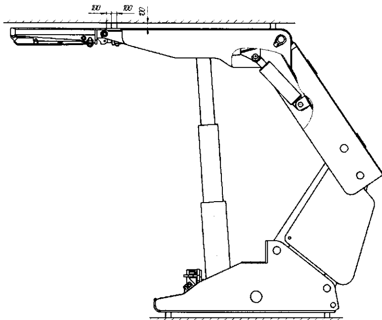
Рис. 1. Установка секции крени на испытательном стенде
