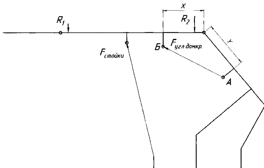
Рис. 2. Схема приложения сил к секции крепи
