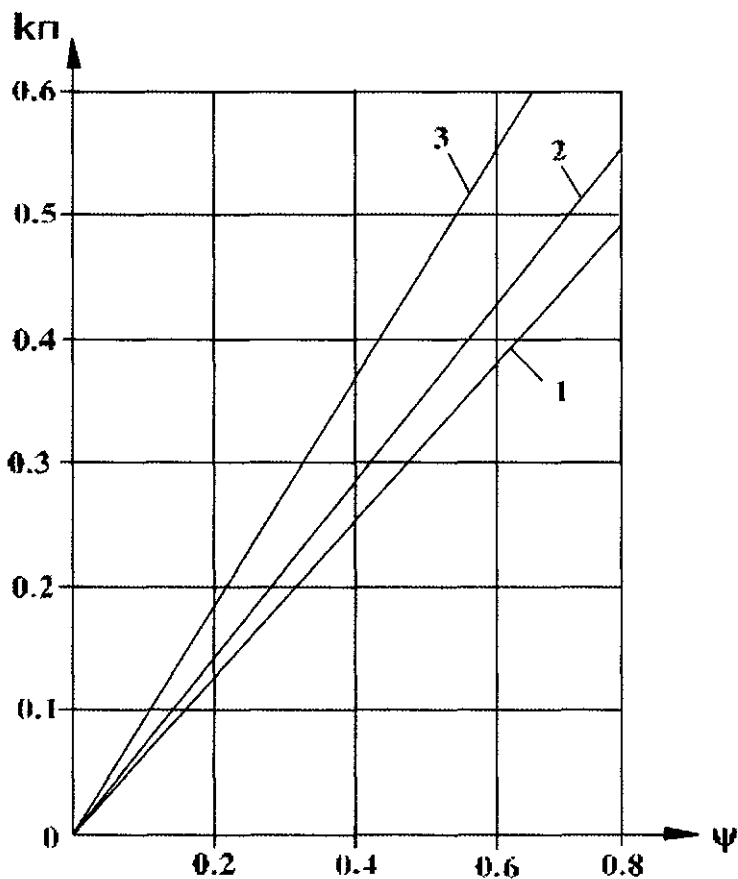
Зависимость коэффициента производительности горизонтального шнека от коэффициента заполнения при транспортировании песка (1), глины (2) и угля (3)
