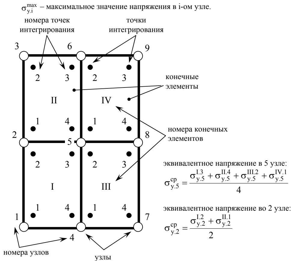
Рис. 1. Схема определения показателя плотности конечно-элементной сетки
