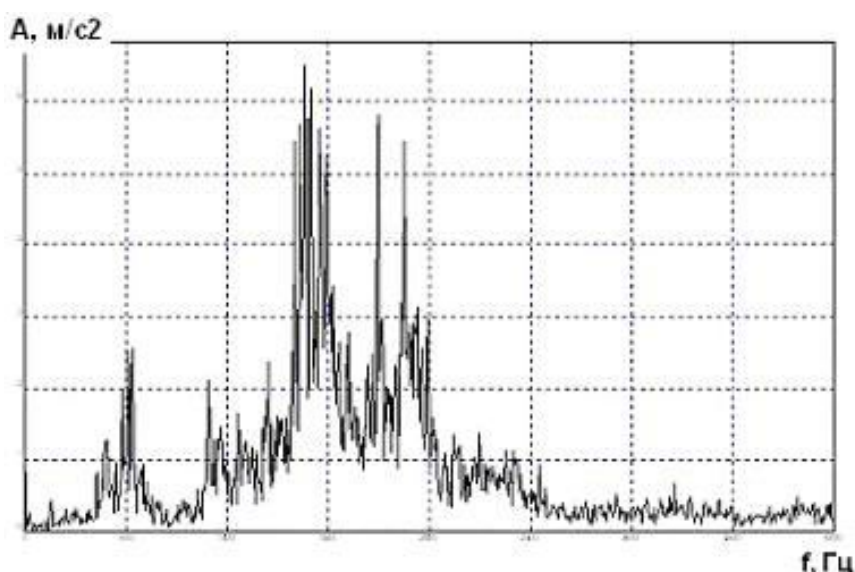
Рис. 3. Развитие дефекта коренного подшипника дизельного двигателя бурового станка DML
