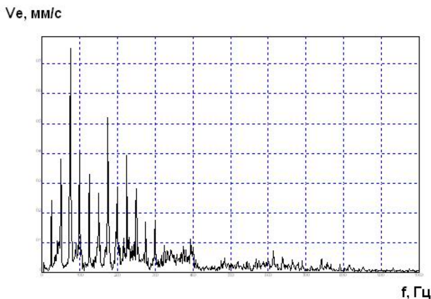
Рис. 2. Расцентровка дизельного двигателя с компрессором, нарушение жесткости системы
