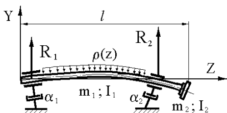
Рис. 1. Схема вала ротора привоного двигателя с опорами на подшипники скольжения
