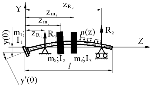
Рис. 3. Расчетная схема вала ротора вентилятора
