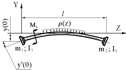
Рис. 2. К выводу уравнения колебаний трансмиссионного вала
