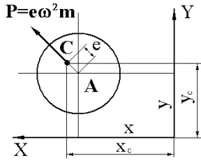
Рис. 4. Схема координатных осей вращающегося неуравновешенного ротора
