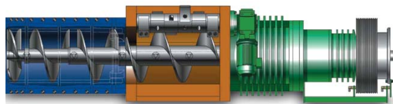
Рис. 1. Машина Futura II E56a/50 для производства окускованного топлива работающая по принципу шнекового пресса
