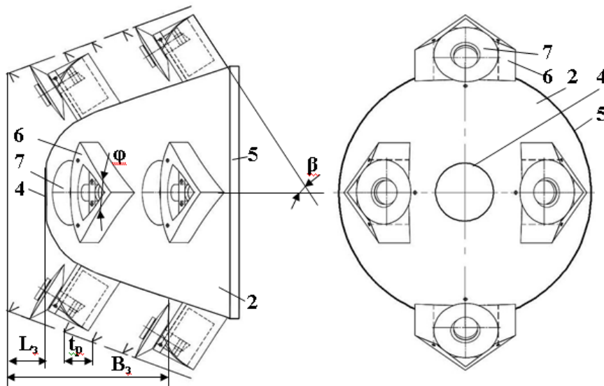
Рис. 2. Первый вариант исполнения унифицированной коронки
