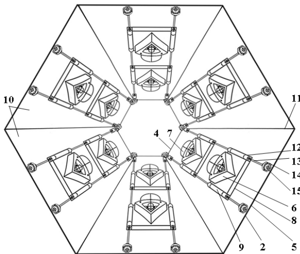
Рис. 3. Второй вариант исполнения унифицированной коронки
