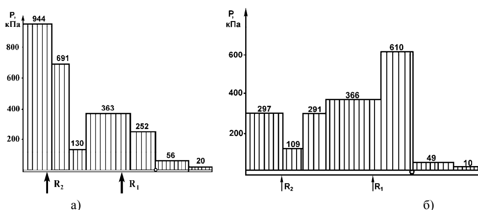
Рис. 1. Характер распределения сопротивления крепи по длине перекрытия: а) при подходе к заколу основной кровли; б) после прохода закола основной кровли (R 1 и R 2 – соответственно усилия забойной и завальной гидростоек)
