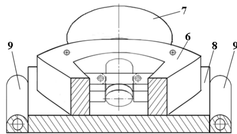
Рис. 4. Сменный разрушающе-погрузочный узел с дисковым инструментом
