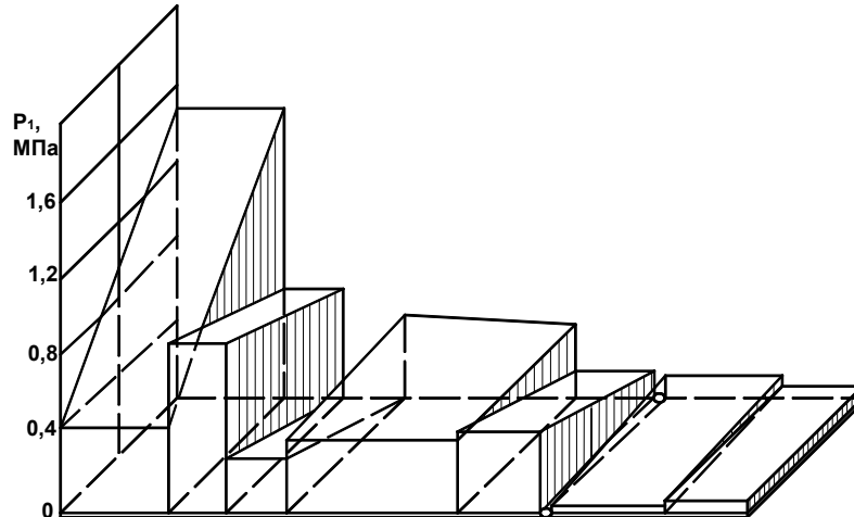
Рис. 2. Распределение сопротивления крепи по площади перекрытия при подходе к заколу основной кровли
