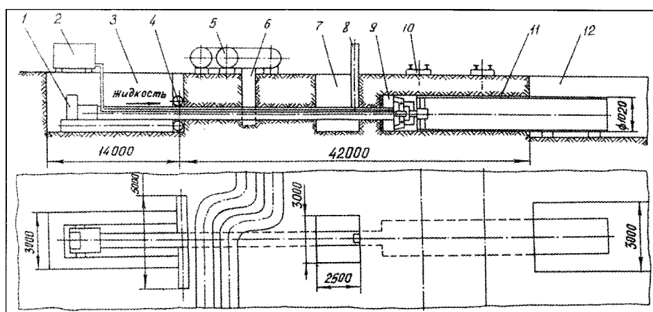
Рис. 2. Схема проведения горизонтальной скважины бурови́ковой машиной с электроприводом и увлажнением продуктов разрушения для газопровода в г.Новокузнецке: 1 — бурови́ковая установка; 2 — емкость в жидкостью; 3 — рабочий котлован; 4 — якорь; 5 — теплотрасса; 6 — бетонная опора; 7 — промежуточный котлован; 8 — свая; 9 — расширитель обратного хода; 10 — железнодорожный путь; 11 — кожух; 12 — приемный котлован
