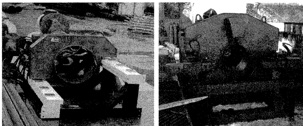
Рис. 1. а — бурови́ковая машина с электрическим приводом; б — бурови́ковая машина с гидравлическим приводом
