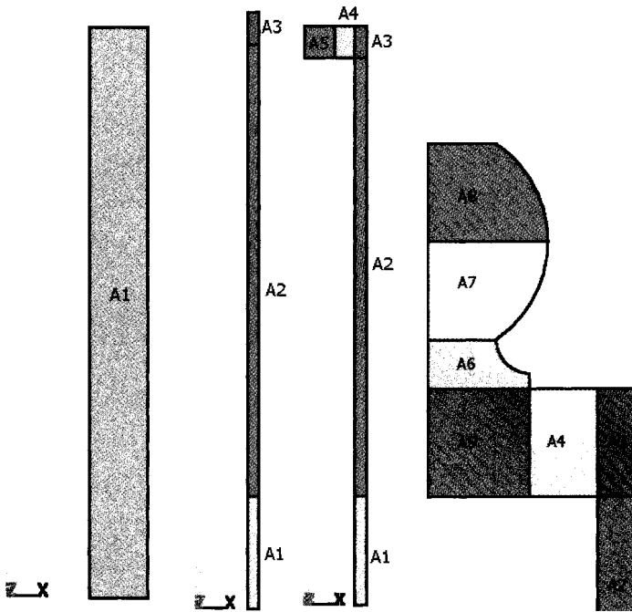
Рис. 3. Порядок построения геометрической модели цилиндра
