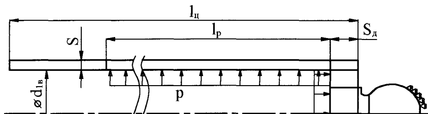
Рис. 2. Геометрическая модель цилиндра
