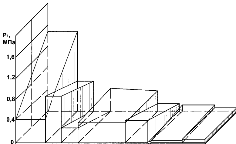
Рис. 3. Распределение сопротивления крепи по площади перекрытия при подходе к заколу основной кровли
