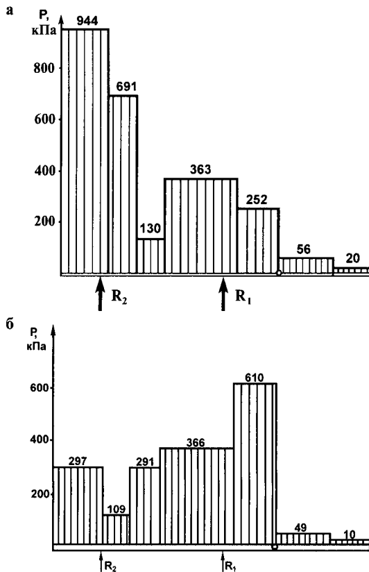
Рис. 1. Характер распределения сопротивления крепи по длине перекрытия: а) при подходе к заколу основной кровли; б) после прохода закола основной кровли ( R_1 и R_2 — соответственно усилия забойной и завальной гидростоек)
