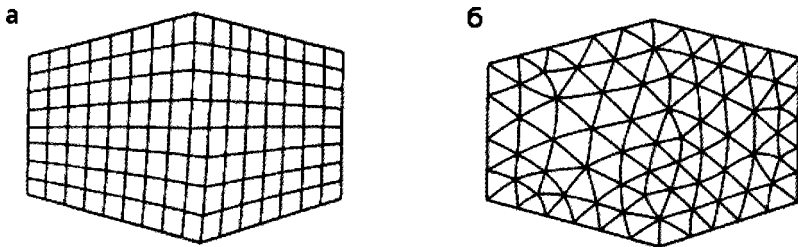
Рис. 1. Регулярная (а) и свободная (б) сетки конечных элементов
