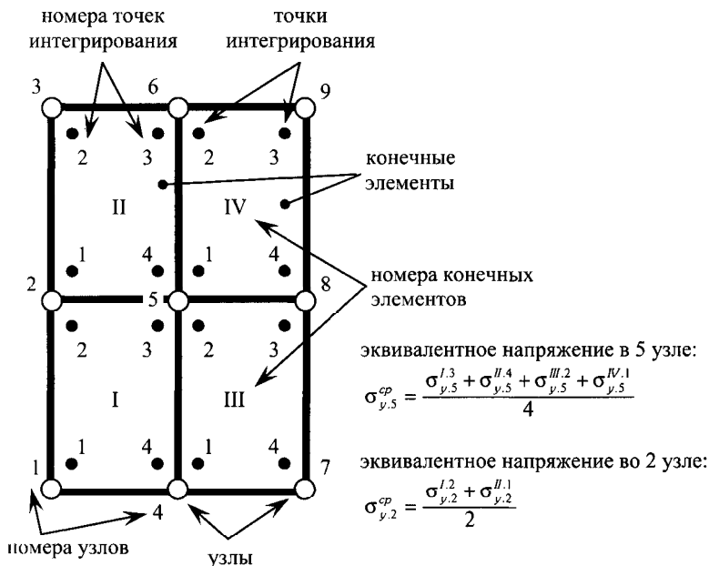
Рис. 1. Схема определения показателя плотности конечно-элементной сетки модели
