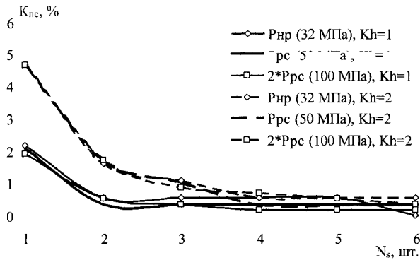
Рис. 2. Показатель плотности сетки конечных элементов для цилиндра гидростойки М130 при различных давлениях жидкости ( P ) в рабочей полости, формах конечных элементов ( K_h ) и количествах элементов по толщине стенки цилиндра ( N_s )
