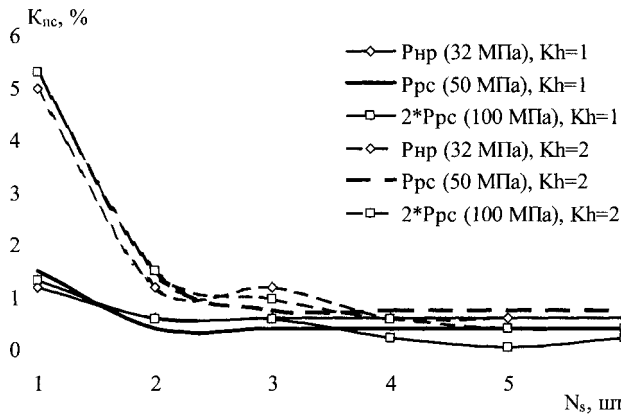
Рис. 3. Показатель плотности сетки конечных элементов для цилиндра гидростойки ОКП70 при различных давлениях жидкости ( P ) в рабочей полости, формах конечных элементов ( K_h ) и количествах элементов по толщине стенки цилиндра ( N_s )
