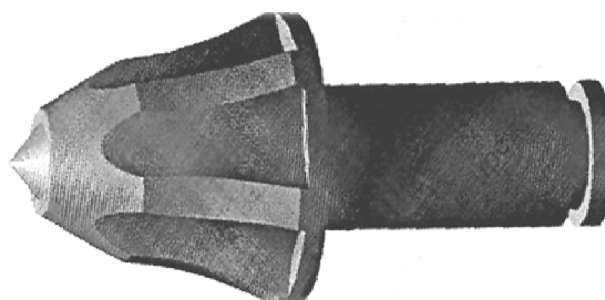
Рис. 2. Конструкция ТПР с ребрами жесткости.
