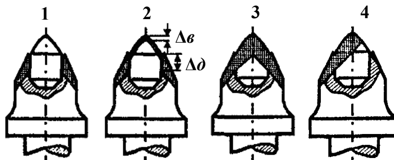
Рис. 1. Формы износа поворотных резцов
