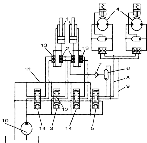
Рис. 3. Фрагмент № 3 гидросхемы
