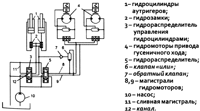
Рис. 2. Фрагмент № 2 гидросхемы комбайна
