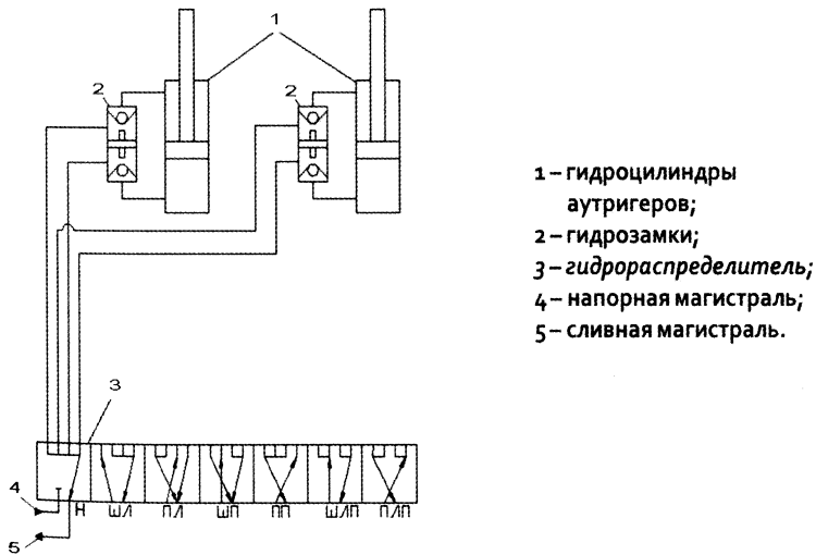
Рис. 1. Фрагмент № 1 гидросхемы комбайна
