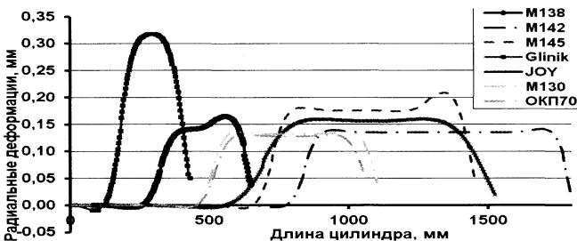
Рис. 1. Радиальные деформации по длине рабочего цилиндра гидростоек механизированных крепей при раздвижности l_p = (2/3)l_p^{\max} при P = 50 МПа
