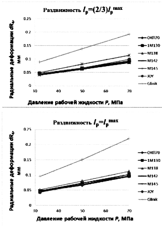
Рис. 3. Изменение радиальных деформаций ( dR_4 ) гидростоек механизированных крепей от давления рабочей жидкости ( P ) при раздвижностях ( l_p )
