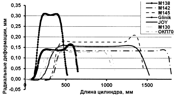
Рис. 2. Радиальные деформации по длине рабочего цилиндра гидростоек механизированных крепей при раздвижности l_p = l_p^{\max} при P = 50 МПа
