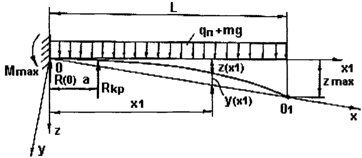
Рис. 3. Расчетная схема определения прогибов блока основной кровли в период, предшествующий проявлению осадки
