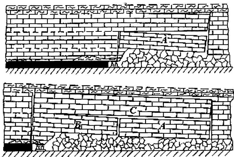
Рис. 1. Характер деформации подработанной толщи при двустадийном проявлении вторичных осадок
