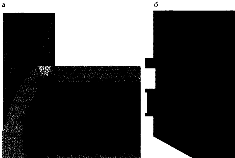
Рис. 2. Разбиение модели на сетку конечных элементов: а — цилиндр гидростойки; б — шток первой ступени
