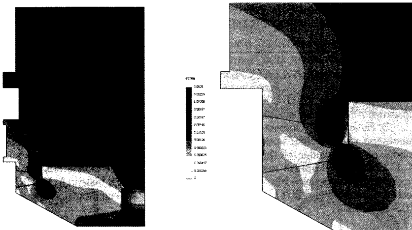
Рис. 8. Распределение деформаций в штоке первой ступени
