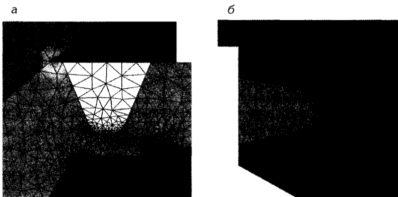
Рис. 3. Уплотнение сетки конечных элементов в области сварного шва: а — цилиндр гидростойки; б — шток первой ступени
