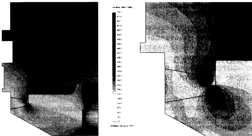
Рис. 7. Распределение эквивалентных напряжений по критерию Мизеса в штоке первой ступени
