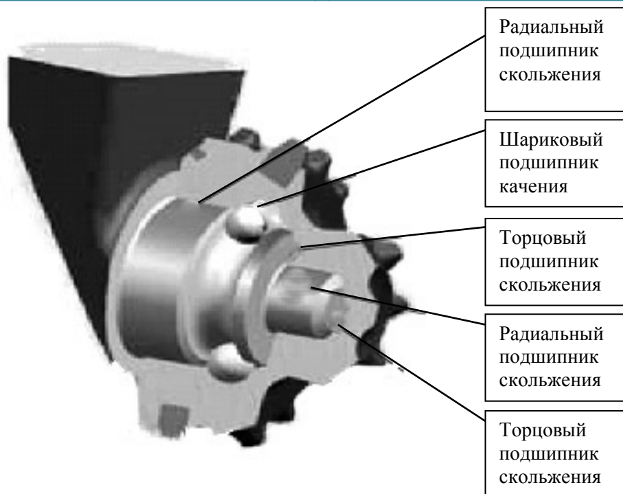
Рис.1 Конструкция опоры на подшипниках скольжения серийных долот
