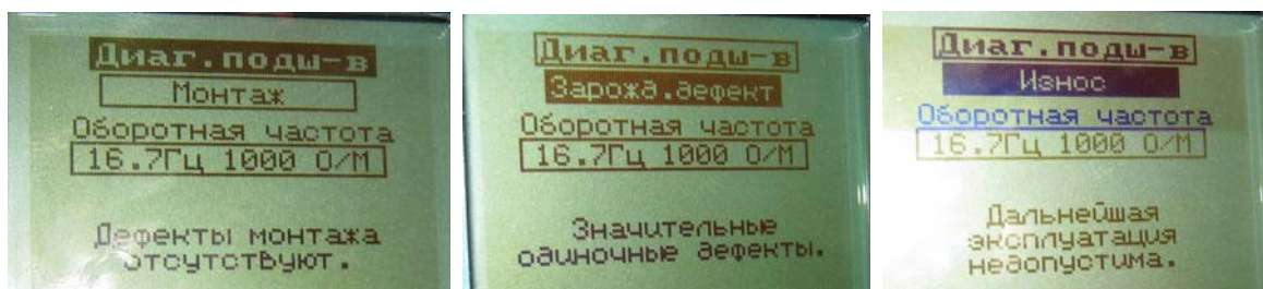
Рис. 5. Диагностика подшипника синхронного двигателя: а) – проверка монтажа, б) – наличие зарождающихся дефектов, в) – износ.
