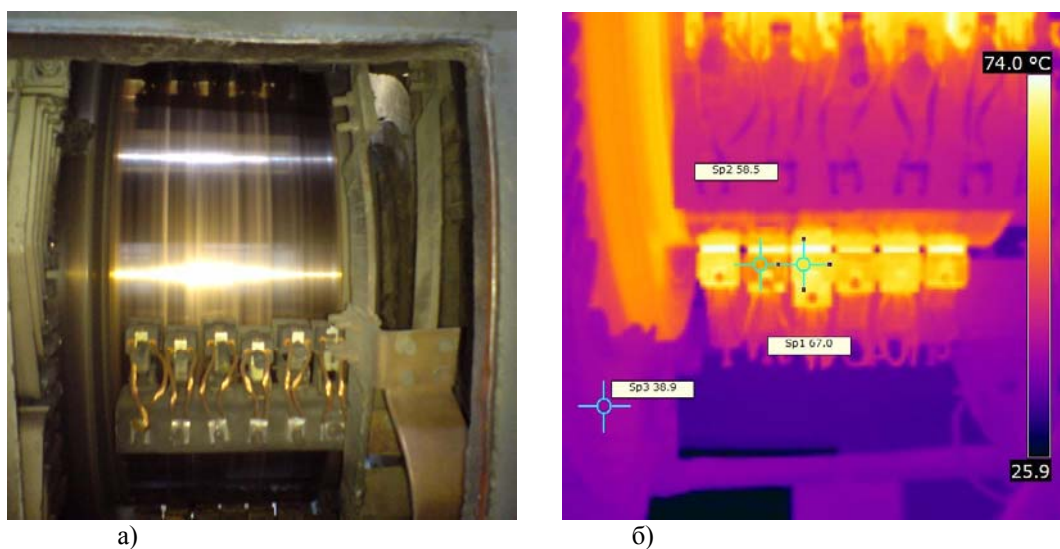
Рис. 2. Щеточно-коллекторный узел генератора напора экскаватора ЭШ-10/70: а) фото, б) инфракрасный снимок (разность температур в 9,5°С на щетках говорит о их неравномерном прилегании к коллектору)
