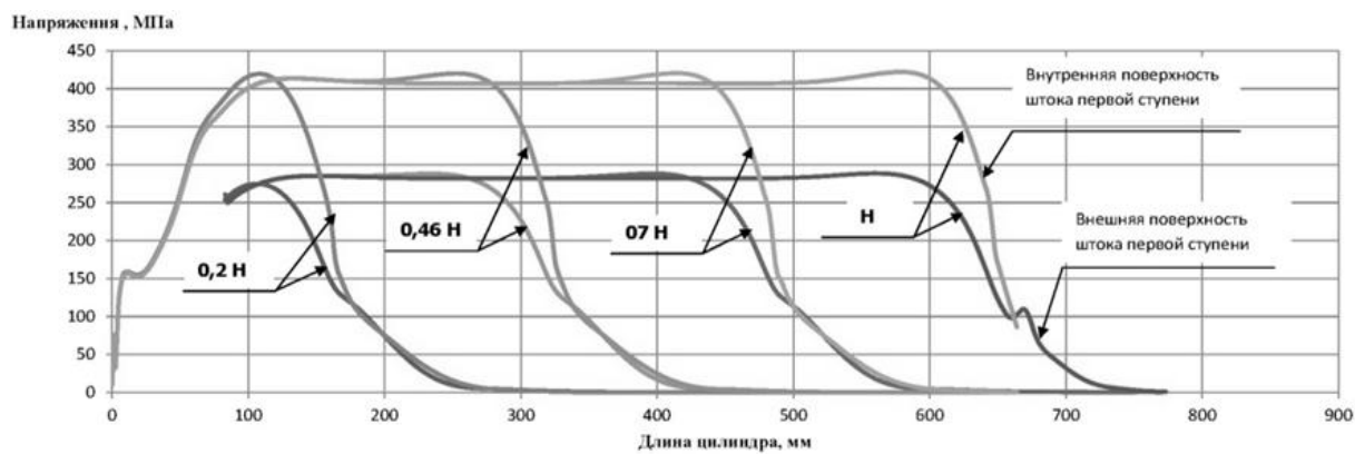
Рисунок 3 - Эквивалентные напряжения по критерию Мизеса для цилиндра
