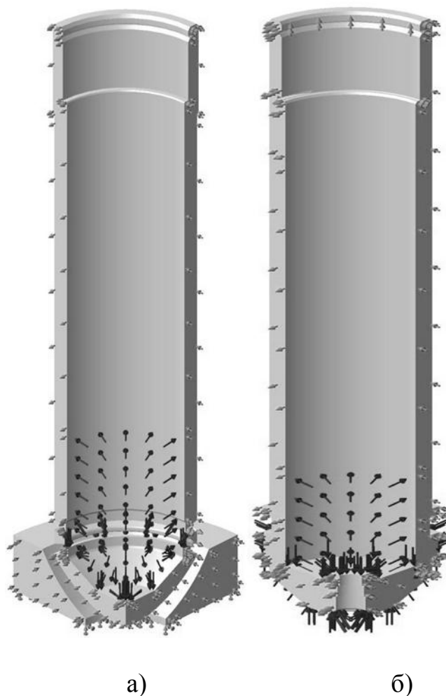
Рисунок 2 - Исследуемые части гидравлической стойки с приложенной нагрузкой и граничными условиями (а - шток первой ступени, б - цилиндр гидравлической стойки)
