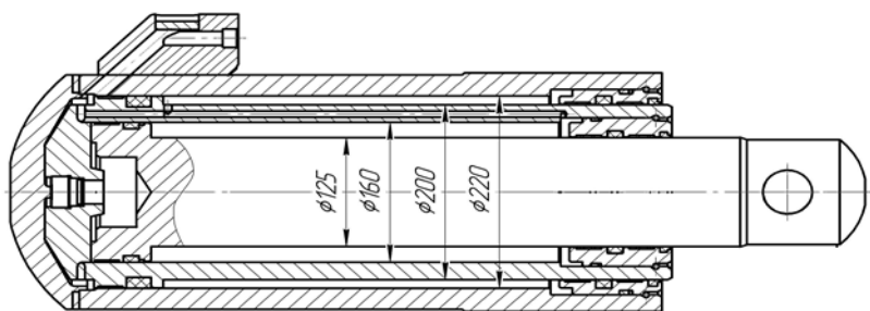
Рисунок 1 - Конструкция рассматриваемой гидравлической стойки
