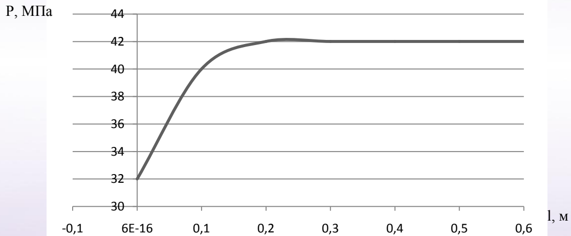
Рисунок 4 – Характеристика гидростоек Дальше осуществляется симуляция работы крепи в шахте (рисунок 5).
