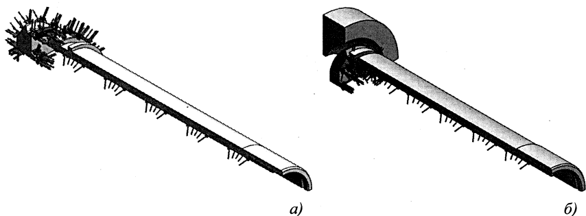
Рис. 2. Исследуемые части гидравлической стойки с приложенной нагрузкой: а – цилиндр гидравлической стойки, б – шток первой ступени
