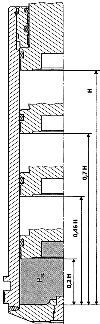
Рис. 6. Радиальные деформации штока первой ступени
