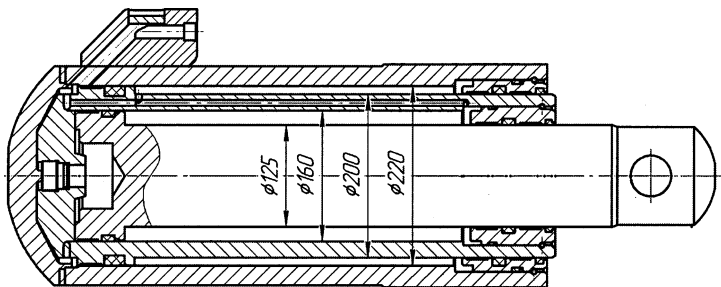
Рис. 1. Конструкция рассматриваемой гидравлической стойки
