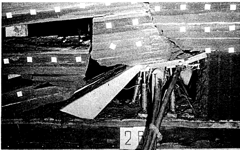
Рис. 2. Прохождение крепию закола кровли
