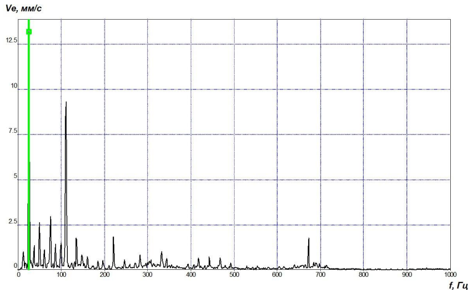
Рис. 5. Малая генераторная группа экскаватора ЭШ 11/70. Недопустимый дисбаланс ротора генератора собственных нужд, ярко выраженное нарушение жесткости системы, ослабление посадки подшипника и нарушение режима его смазки.
