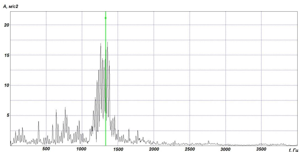
Рис. 1. Развитый дефект подшипника сетевого двигателя экскаватора ЭШ 10/70
