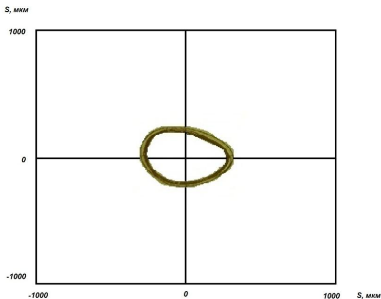
Рис. 4. Орбита синхронного виброакустического сигнала, полученная на сетевом двигателе экскаватора ЭШ 6/45.
