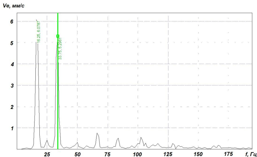
Рис. 3. Дисбаланс ротора генератора поворота, расцентровка с генератором тяги экскаватора ЭШ 15/90.
