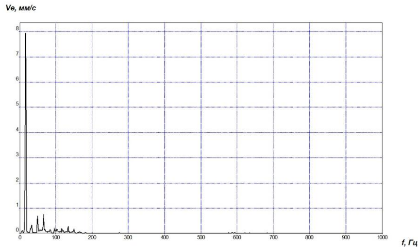
Рис. 2. Преобразовательный агрегат экскаватора ЭШ 13/50. Ярко выраженная расцентровка генераторов поворота и тяги в горизонтальной плоскости.
