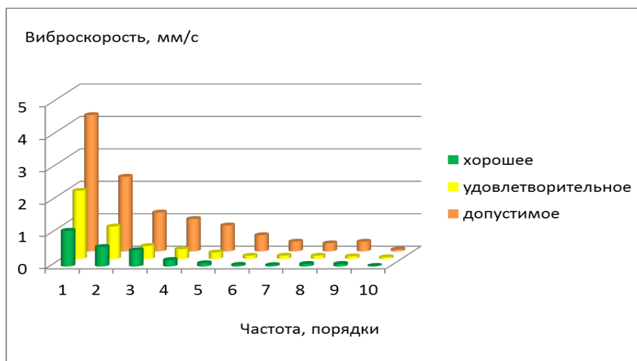
Рис. 2. Пример нормирования состава полигармонической волны вибрации для генераторной группы экскаватора типа ЭШ 10/70.
