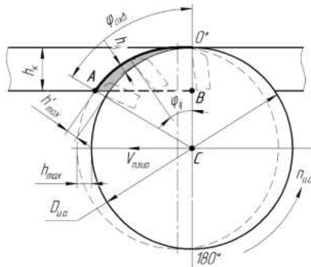
Рисунок 2 – Схема к определению текущего значения глубины стружки на дисковом ЗИО
