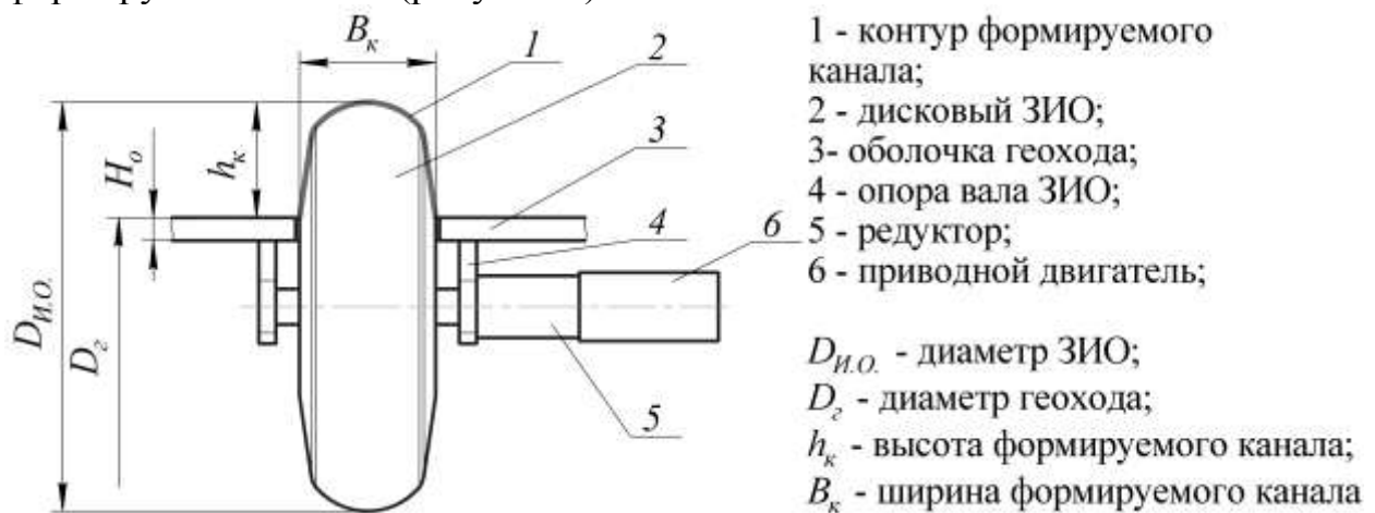
Рисунок 1 – Схема к определению текущего значения глубины стружки на дисковом ЗИО
