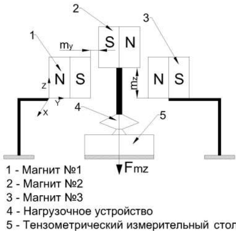
Рис. 1. Схема стенда для испытания
