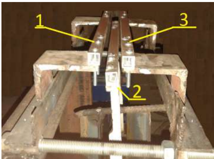
Рис. 2. Экспериментальный стенд магнитного подвеса
