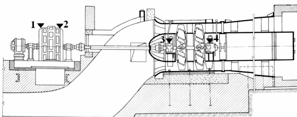
Рис. 1. Контрольные точки измерения вибрации на осевом вентиляторе главного проветривания ВОКД-1,8
