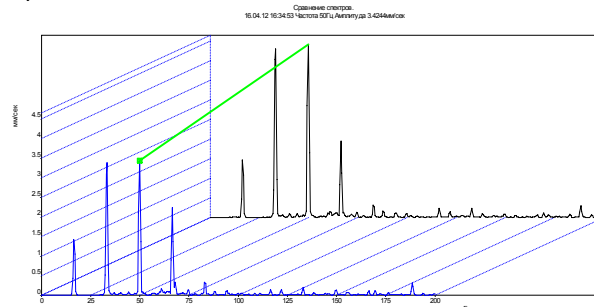
Рис. 3. Сравнение спектров в 3 контрольной
