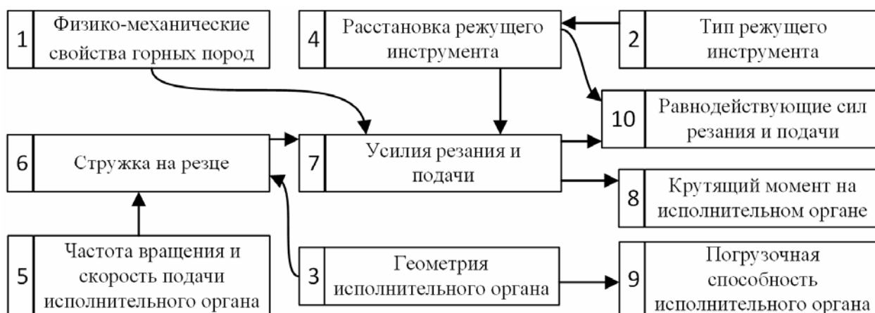
Рисунок 1 – Алгоритм определения параметров режущих исполнительных органов
