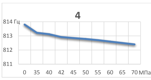
Рис. 4. Изменение модальной частоты 4
