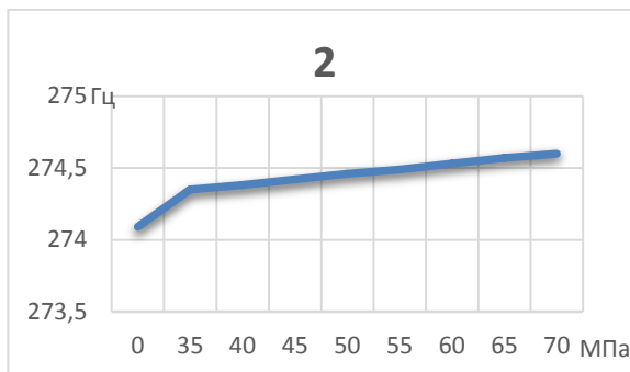
Рис. 2. Изменение модальной частоты 2
